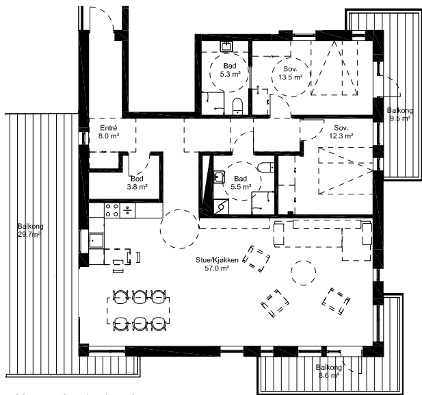
Alternativ planløsning
